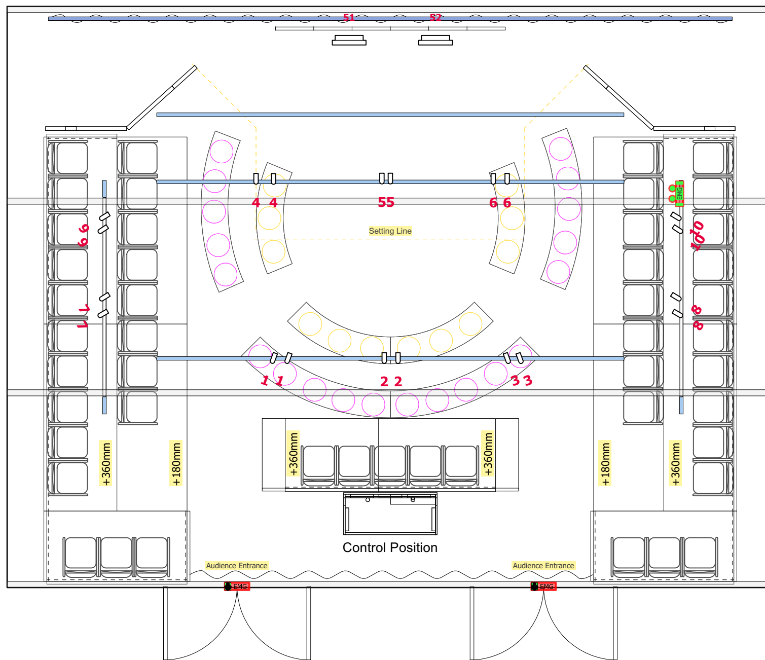
1 Green - Kids Layout Scale: 1:50
