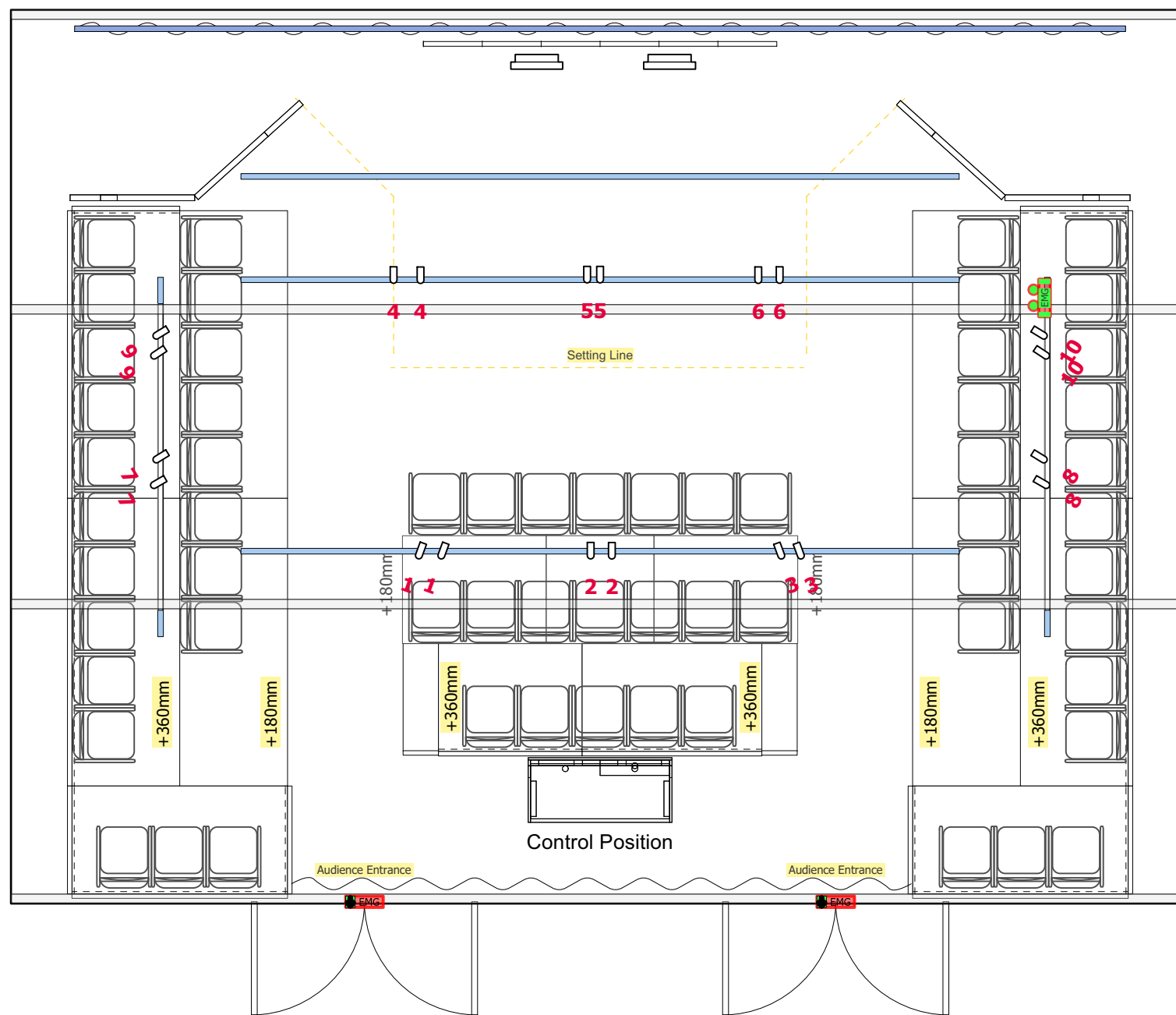
2 Green - Adult Layout Scale: 1:50
